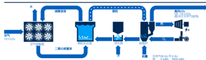
图 23 CARBON ENGINEERING直接空气捕集和封存技术
