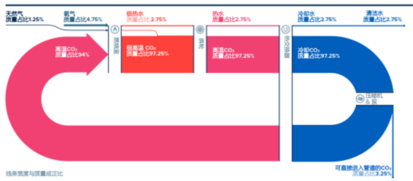
图21 ALLAM-FETVEDT循环工艺流程图 来源：8 Rivers Capital (供图)
