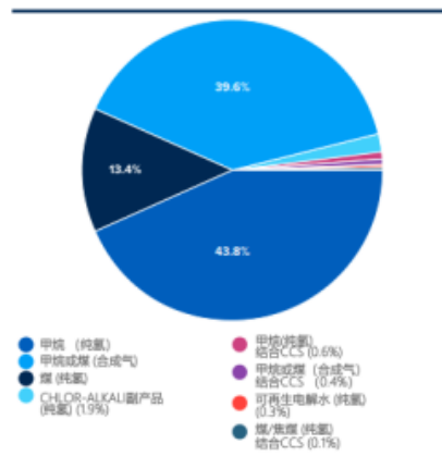
图17 全球不同来源和工艺的制氢比例
