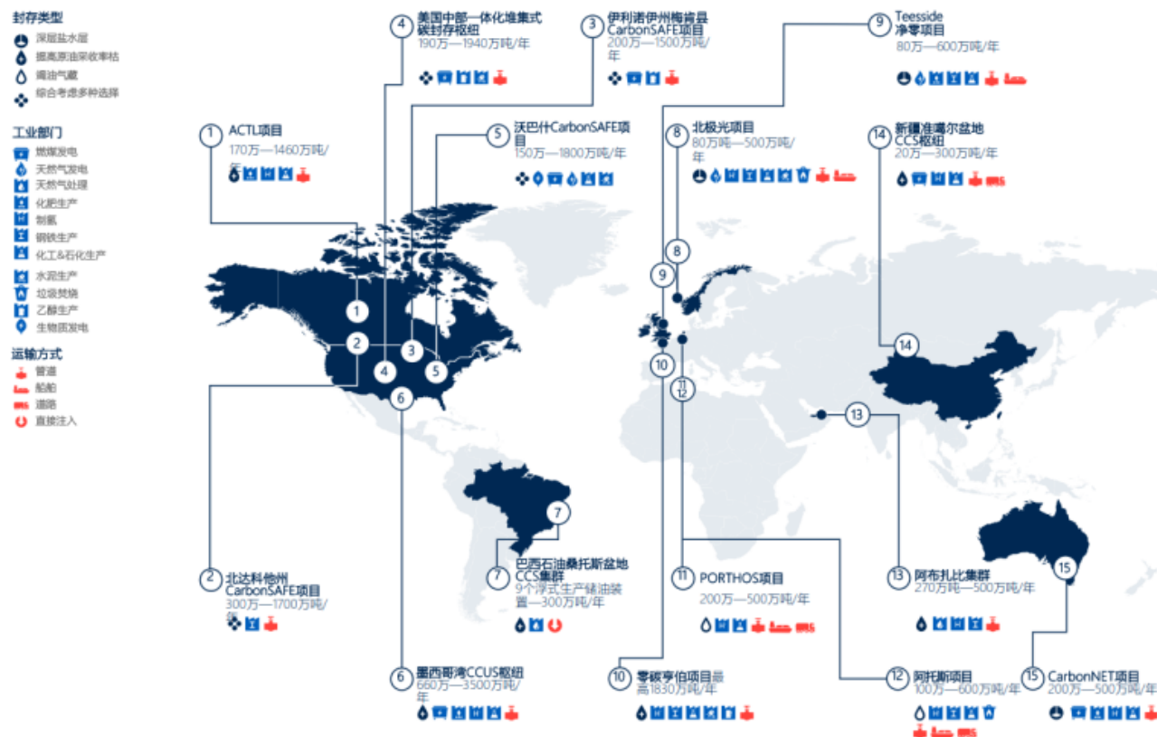
图7 处于运行或开发阶段的枢纽和集群
