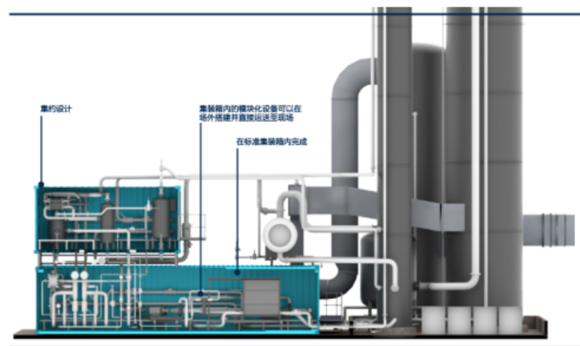
图24 AKER 'JUST CATCH' 模块化碳捕集系统 图片来源：Aker Solutions.
