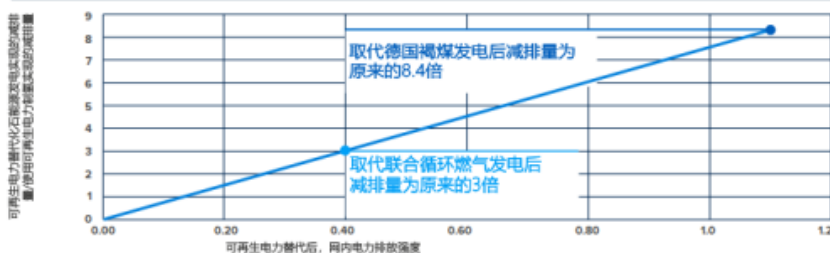
图19 可再生能源替代化石燃料发电实现的减排量远高于使用可再生能源制氢产生的减排量 假设氢气替代天然气燃烧
