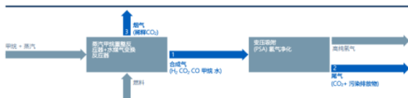
图18 基于SMR的制氢厂工作流程图
