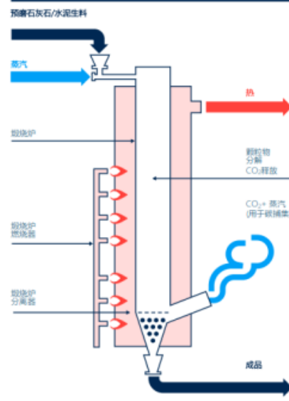
图16 CALIX 先进煅烧反应炉-详图 来源：Calix (提供)
