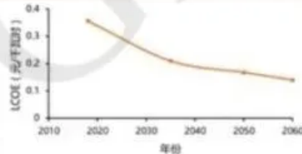
陆上风电度电成本预测
