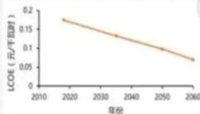
光伏发电度电成本预测
